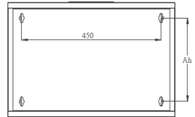
VUE ARRIERE
