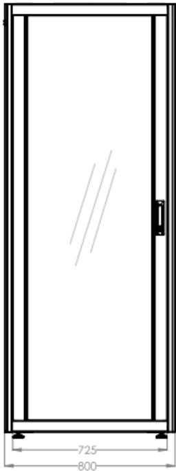
VUE AVANT
