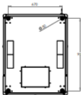
VUE LATERALE
